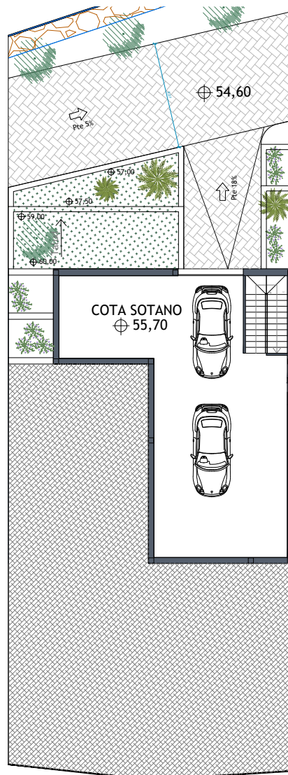
Planta Sótano
