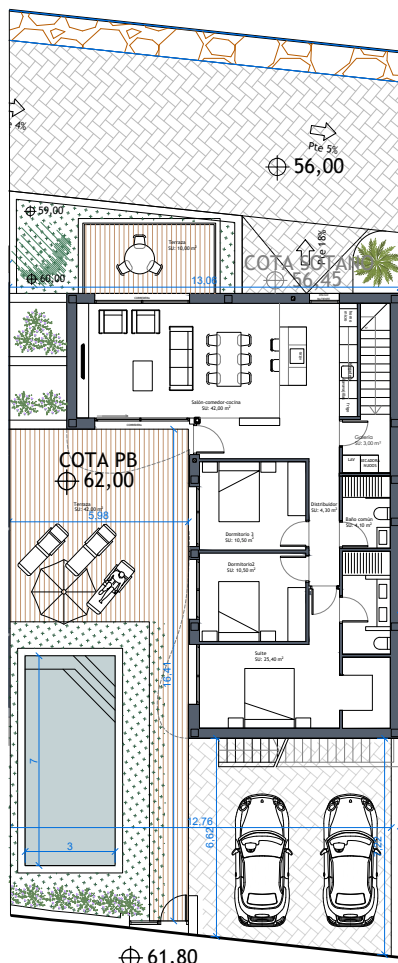
Planta Baja
