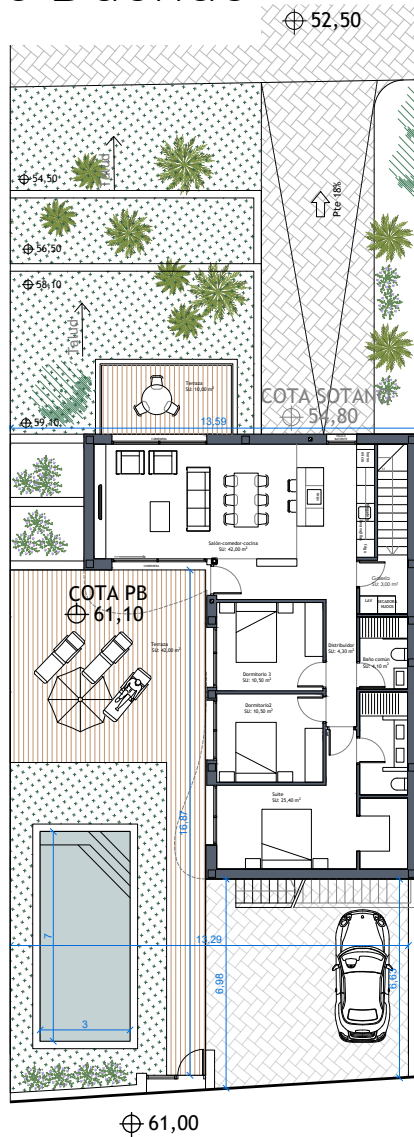
Planta Baja
